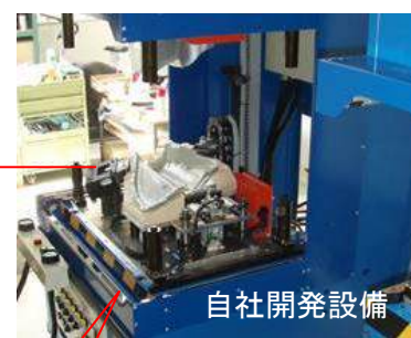
自動車用ドアトリム表皮圧着機
