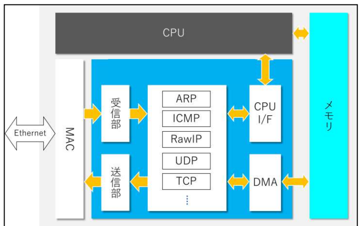
ネットワークアクセラレータ IP の構成 (PTU/Protocol Termination Unit)
